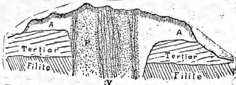
Fi. 3. Profil idealizat prin zăcămintul dela Săcărimb (după B. v. Jnkey)
