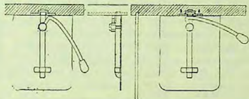
5. Rezemător-fixator pentru cărți, cu manetă.
